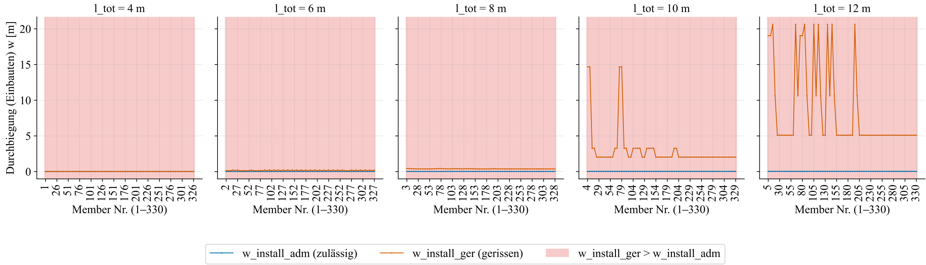
Durchbiegung w_install_adm (zulässig) vs. w_install_ger (Durchbiegung gerissen) je Member, kategorisiert nach Spannweite (Members_rc_rib_simple_V3)
